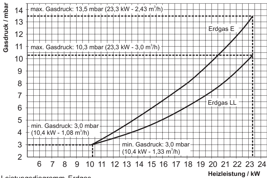
Abb. 5.9 Gas-Leistungsdiagramm Erdgas
