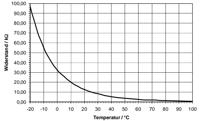
Abb. 4.12 Widerstandskurve
