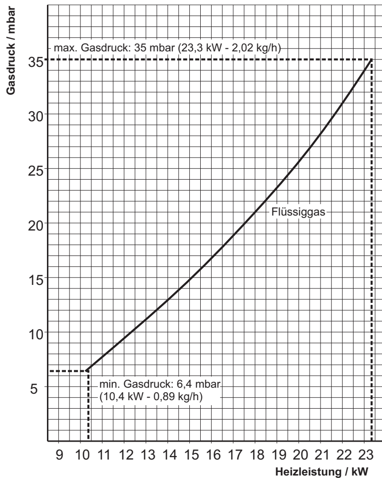
Abb. 5.10 Gas-Leistungsdiagramm Flüssiggas
